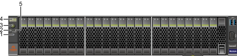
图 2-9 24x2.5 SAS/SATA 直通硬盘配置前面板指示灯和按钮
