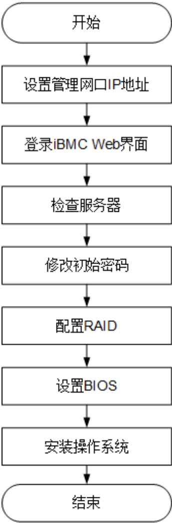
图 5-26 初始配置流程
