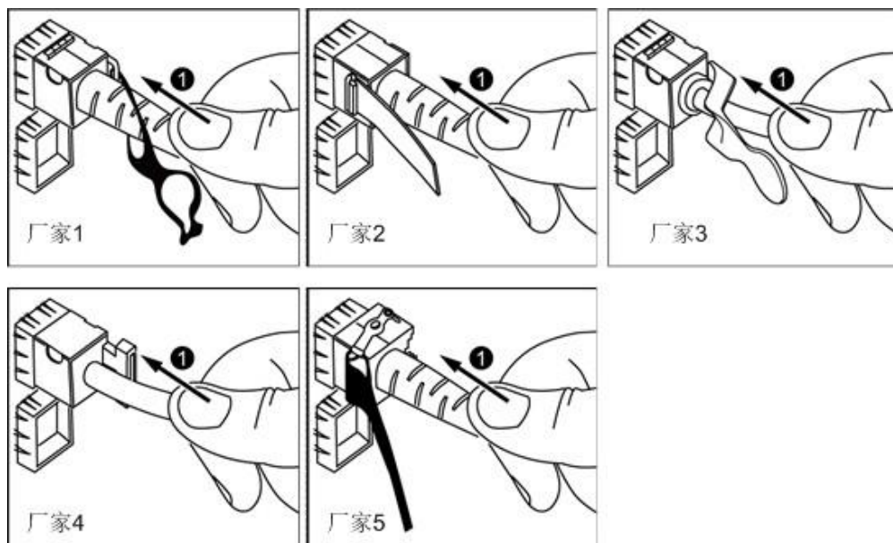
图 5-20 连接 SFP+电缆
