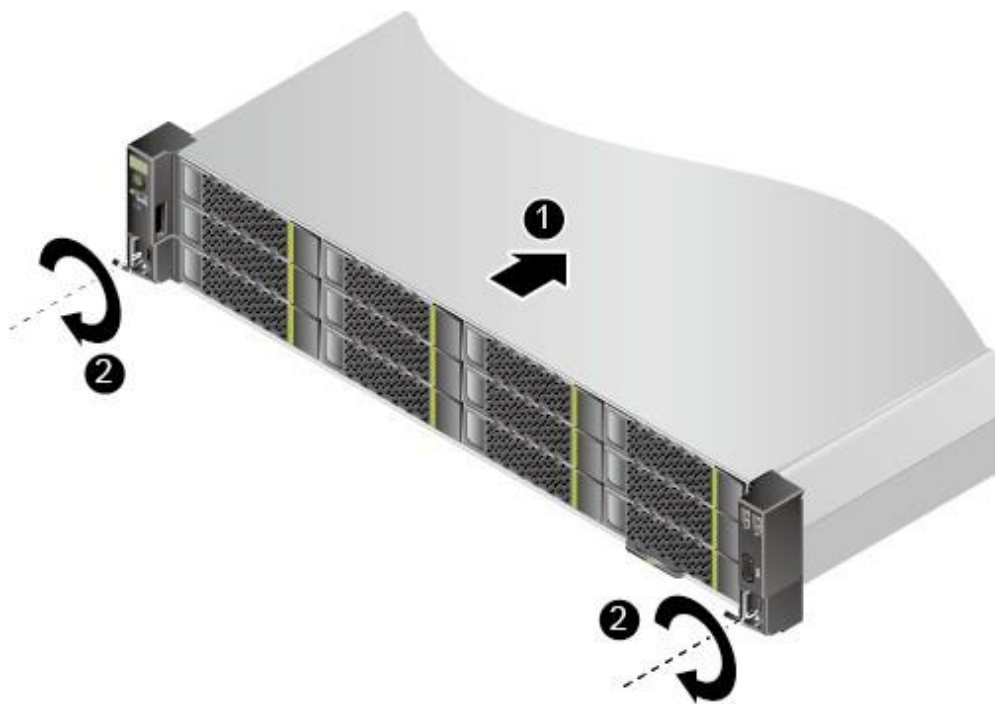
图 5-7 安装服务器
