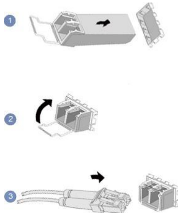
图 5-18 连接光纤
