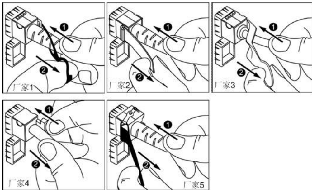
图 5-19 拔出 SFP+电缆
