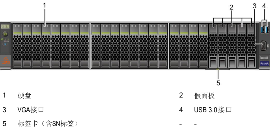
图 2-3 8x2.5 SAS/SATA+12x2.5 NVMe 硬盘配置前面板组件
