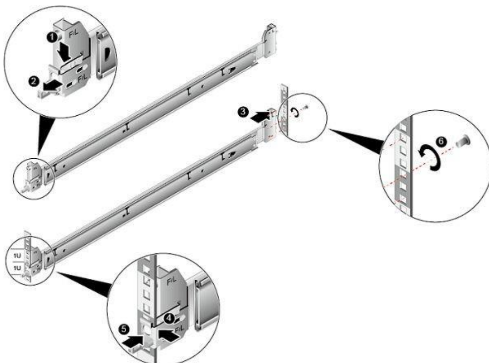
图 5-10 安装抱轨前后端
