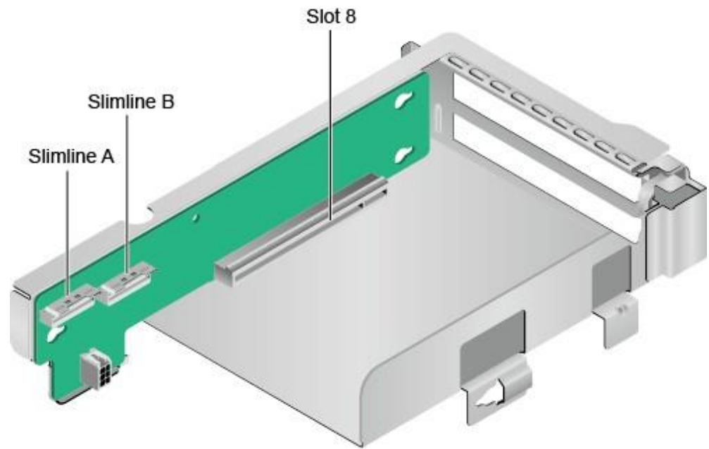
图 2-27 Riser 卡 7（1x16）
