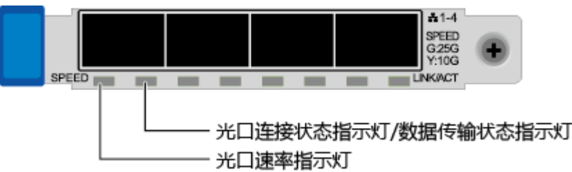
图 2-13 TM280（4x25GE 光口）
