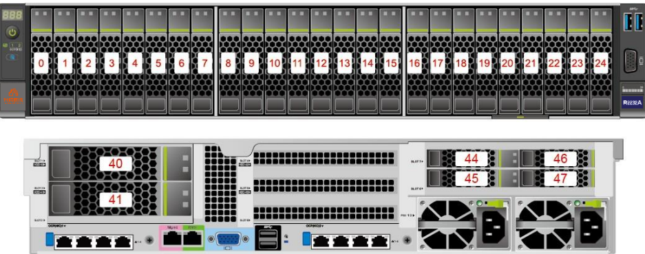
图 2-16 25x2.5 英寸硬盘 EXP 配置硬盘编号
