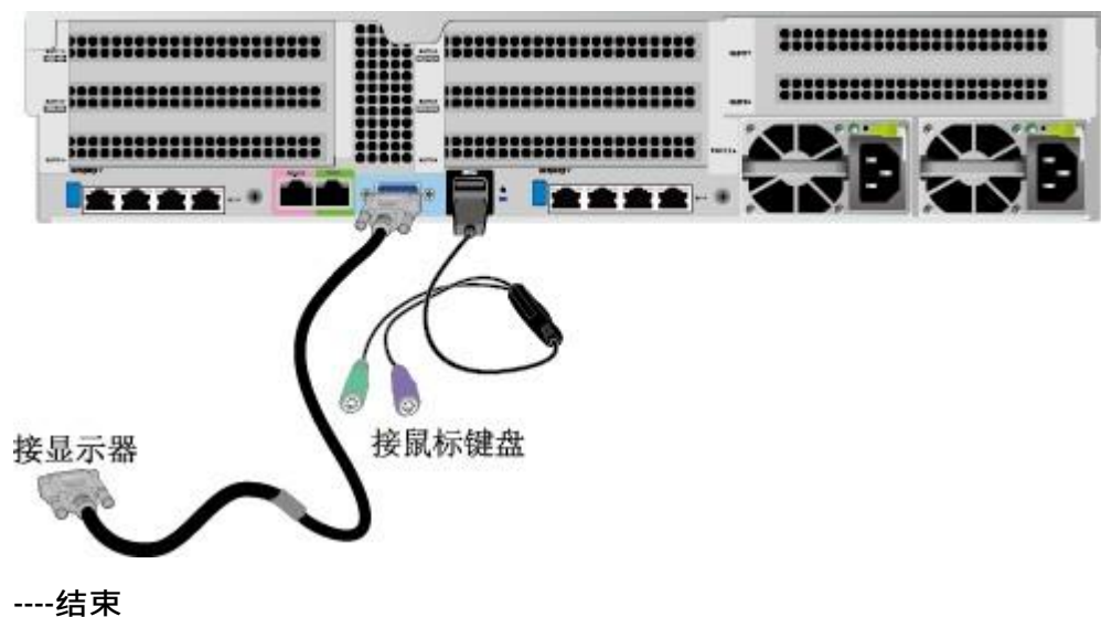
图 5-16 连接 USB 转 PS2 线缆和 VGA 接口
