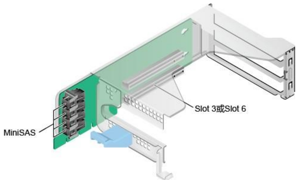
图 2-25 Riser 卡 5 (SAS Riser)
