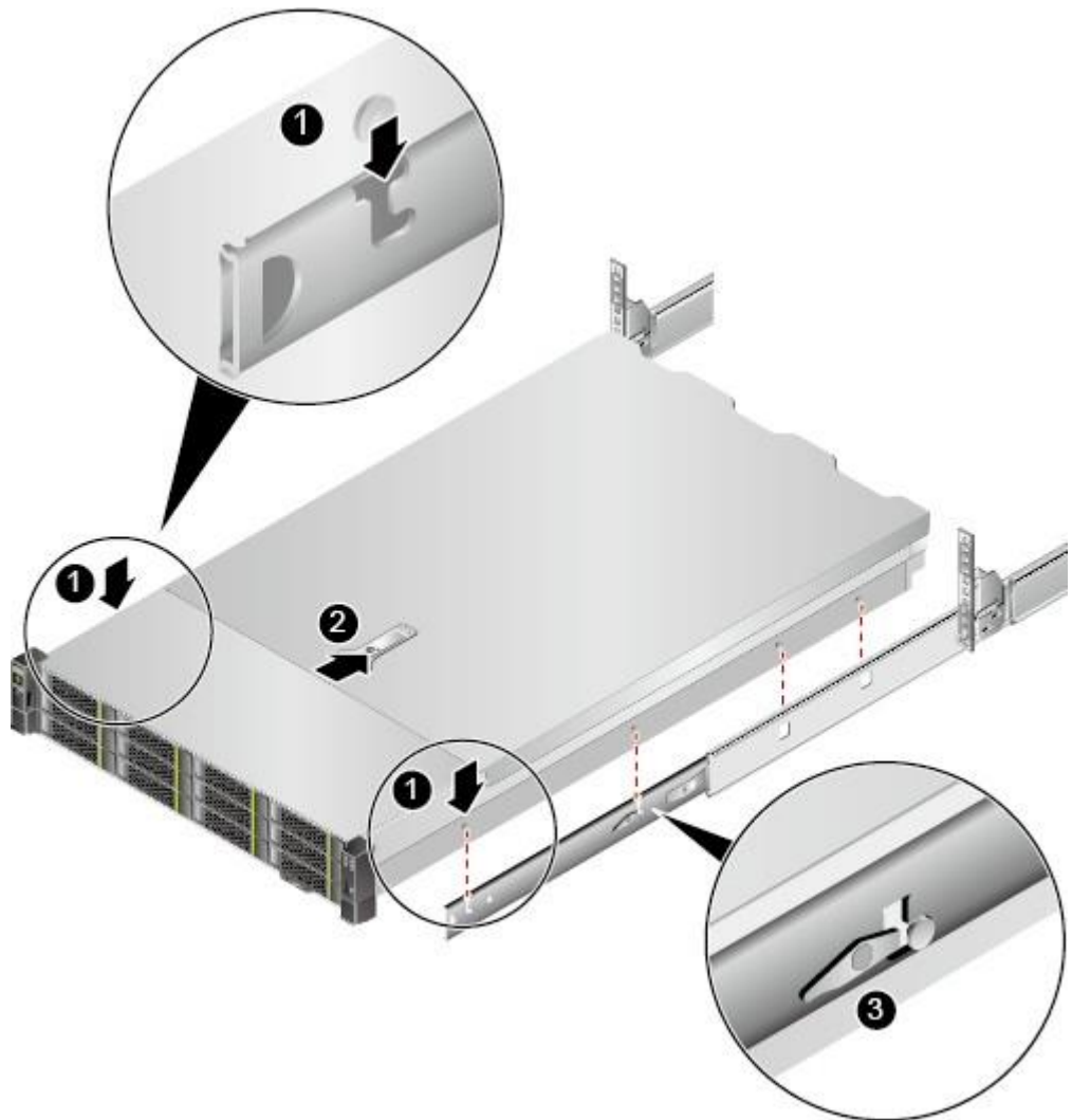
图 5-12 安装服务器
