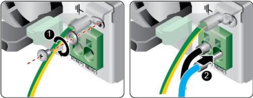
图 5-25 连接线缆
