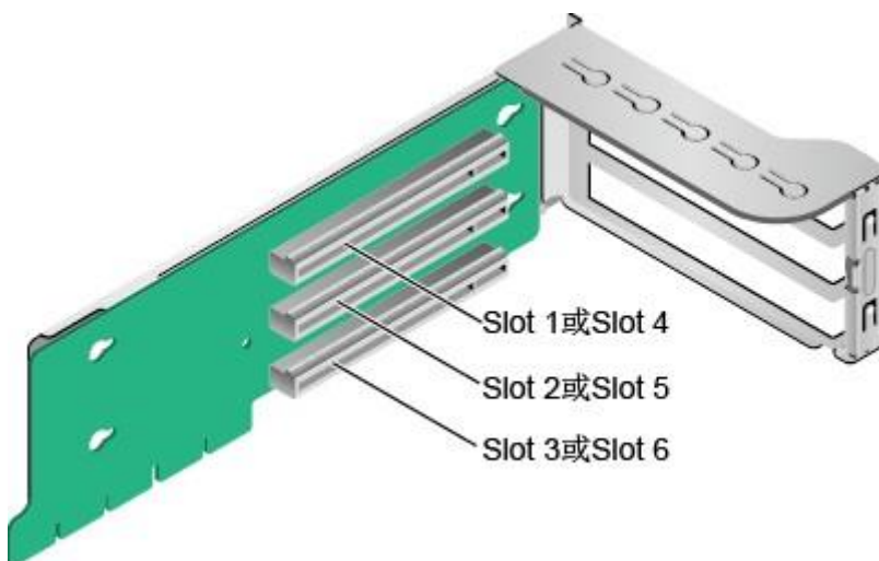
图 2-21 Riser 卡 1（3x8）
