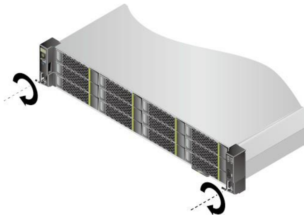
5-14 固定服务器
