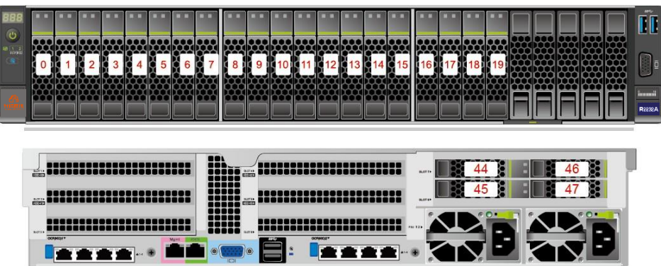
图 2-17 8x2.5 SAS/SATA+12x2.5 NVMe 硬盘配置硬盘编号
