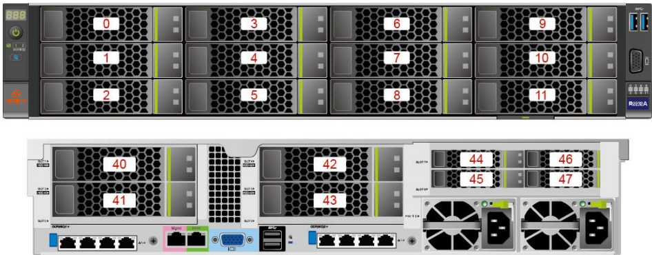
图 2-14 12x3.5 英寸硬盘 EXP 配置硬盘编号
