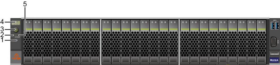
图 2-7 25x2.5 英寸硬盘配置前面板指示灯和按钮
