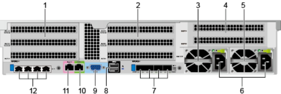
图 2-10 后面板组件
