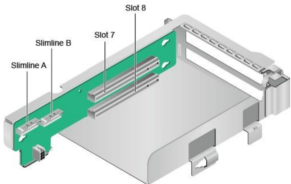
图 2-26 Riser 卡 6 (2x8)
