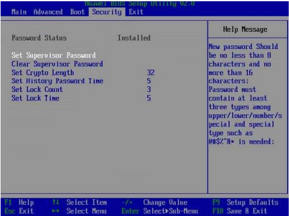
图 5-50 “Security” 界面
