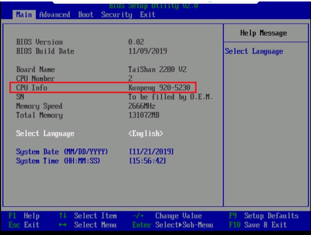
图 8-21 “Main” 界面
