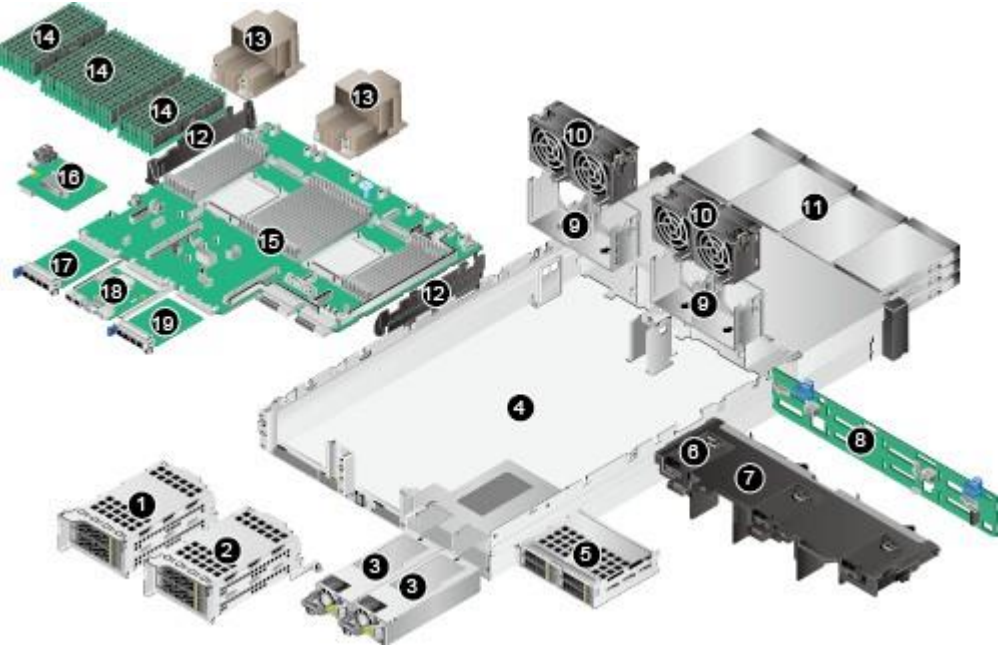
图 1-2 部件（配置鲲鹏 920 7260、5250 或 5230 处理器）
