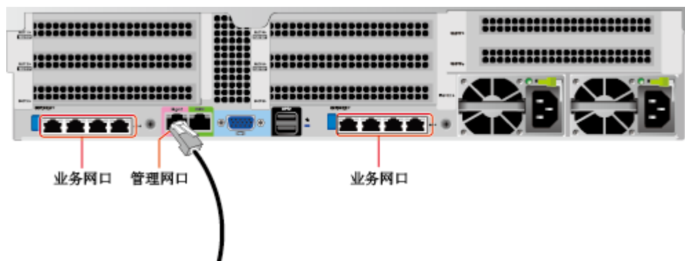
图 5-17 连接网线
