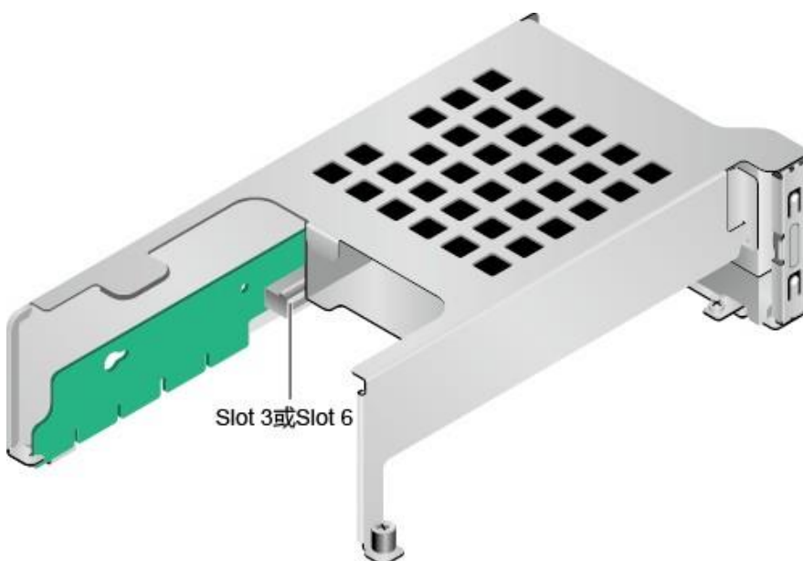
图 2-24 Riser 卡 4（1x16）
