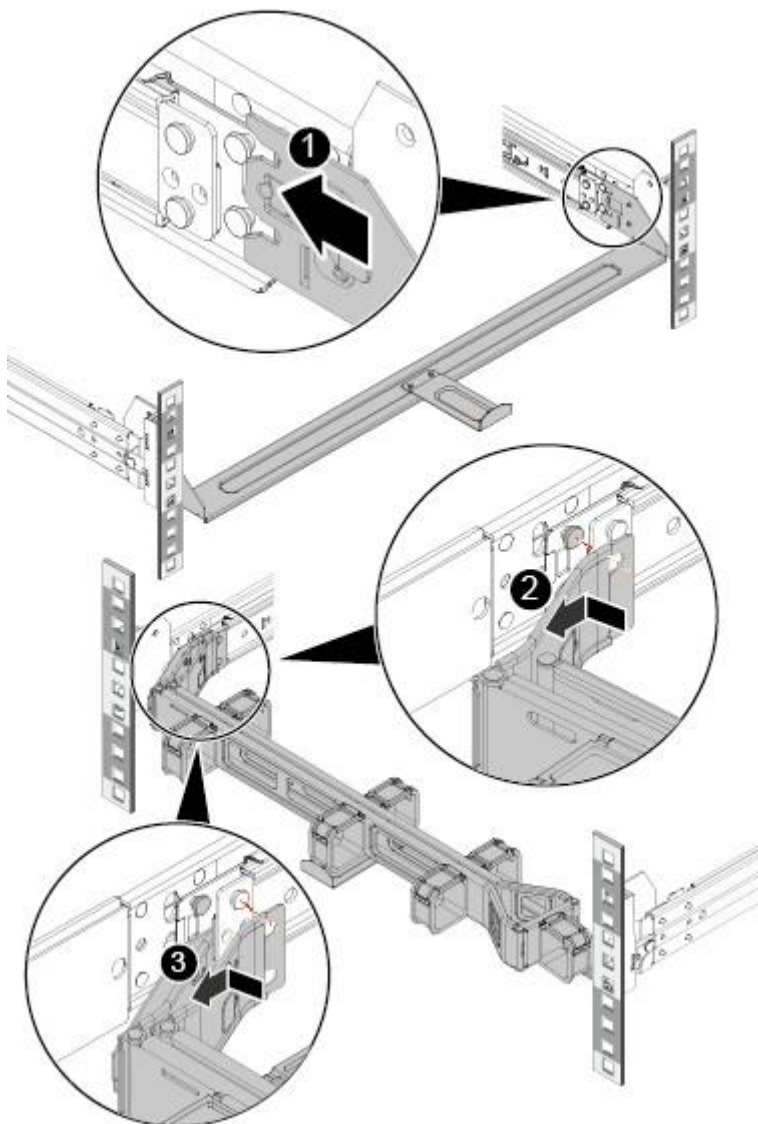
图 5-15 安装理线架
