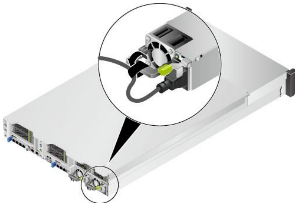
图 5-24 固定电源线缆
