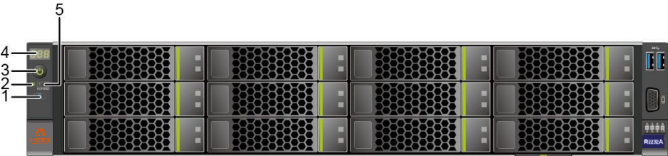
图 2-6 12x3.5 英寸硬盘配置前面板指示灯和按钮
