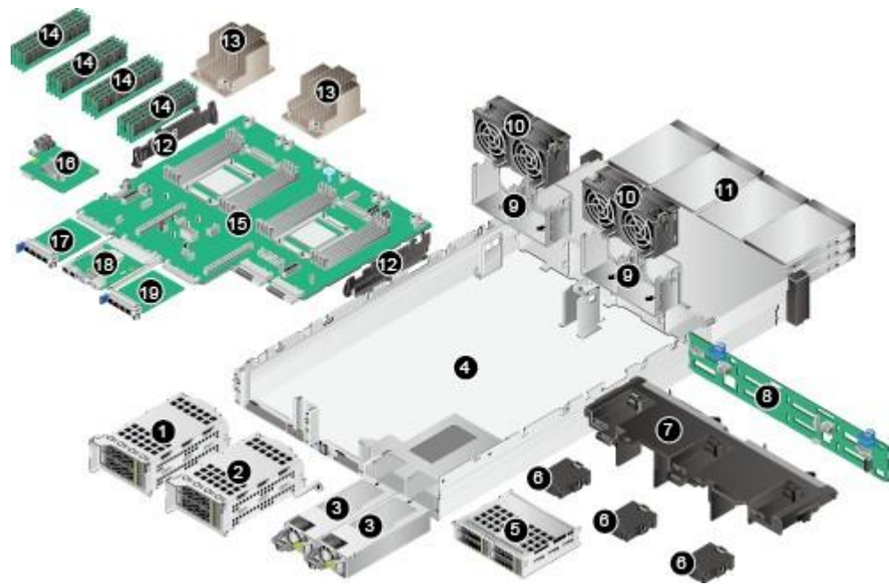
图 1-3 部件（配置鲲鹏 920 5220 或 3210 处理器）
