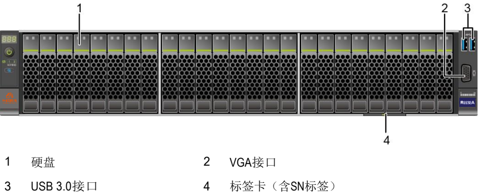
图 2-2 25x2.5 英寸硬盘配置前面板组件
