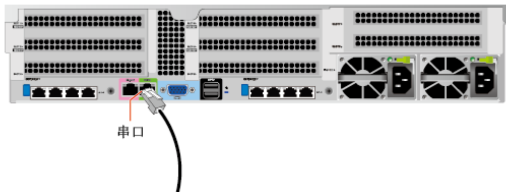
图 5-22 连接串口线缆
