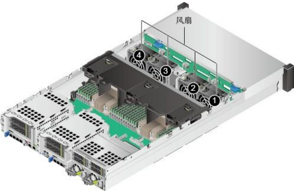
图 2-29 风扇位置图
