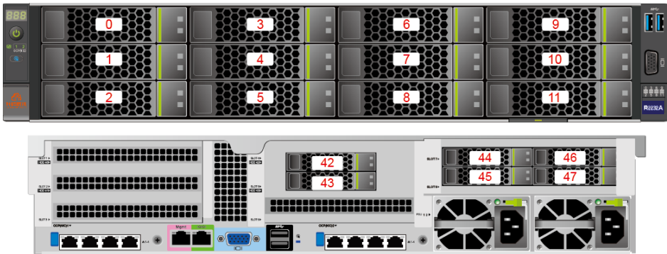
图 2-15 12x3.5 英寸硬盘直通配置
