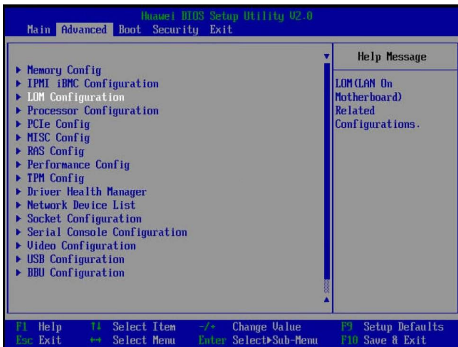
图 5-47 “Advanced” 界面
