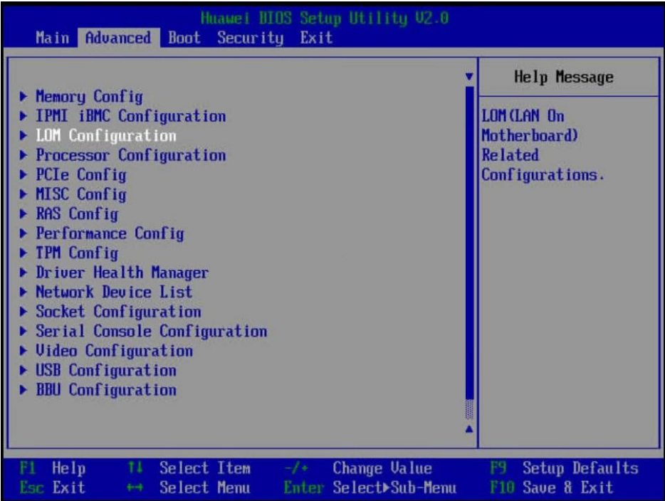
图 5-48 “Advanced” 界面
