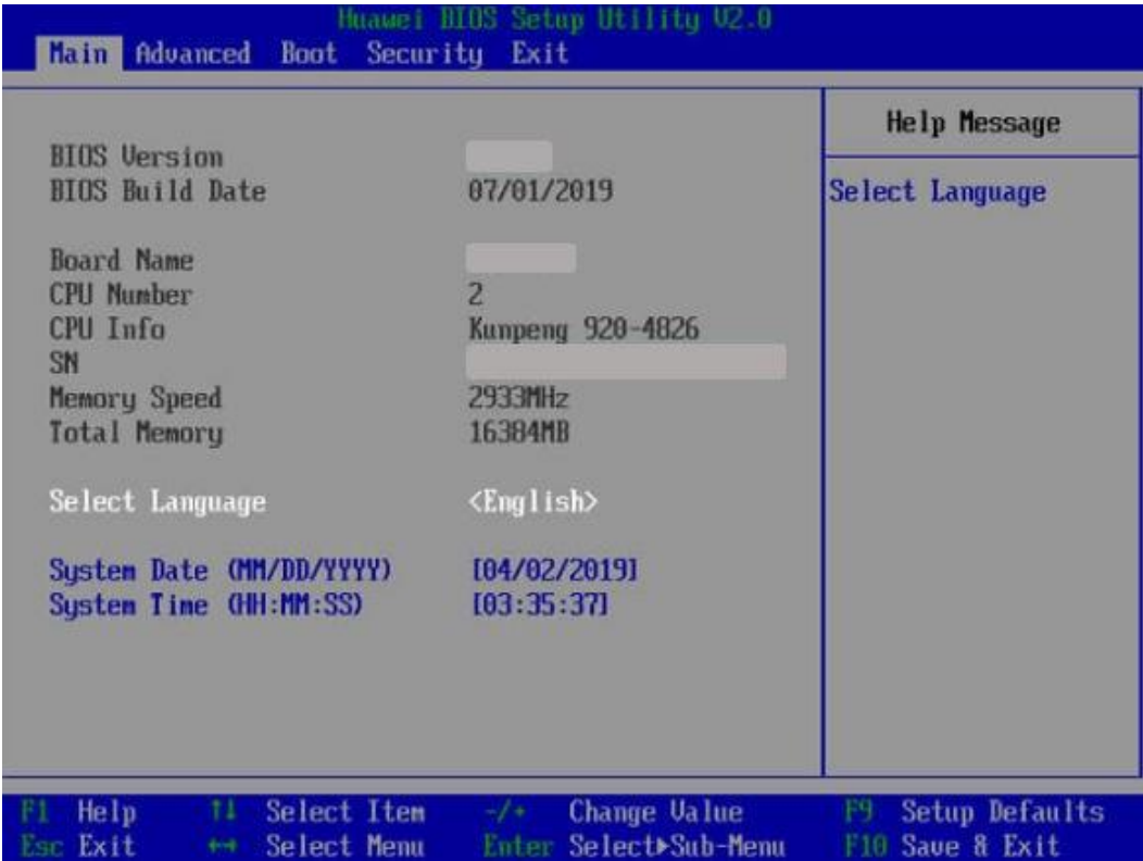
图 5-51 “Main”界面
