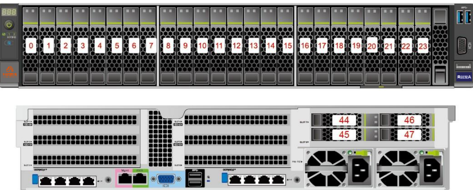
图 2-18 24x2.5 SAS/SATA 直通硬盘配置
