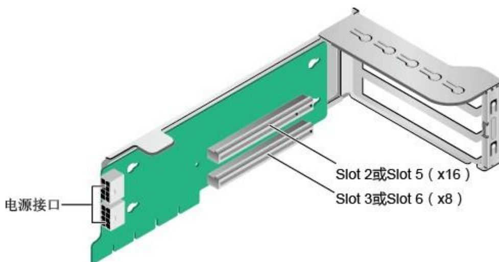
图 2-22 Riser 卡 2（1x8+1x16）
