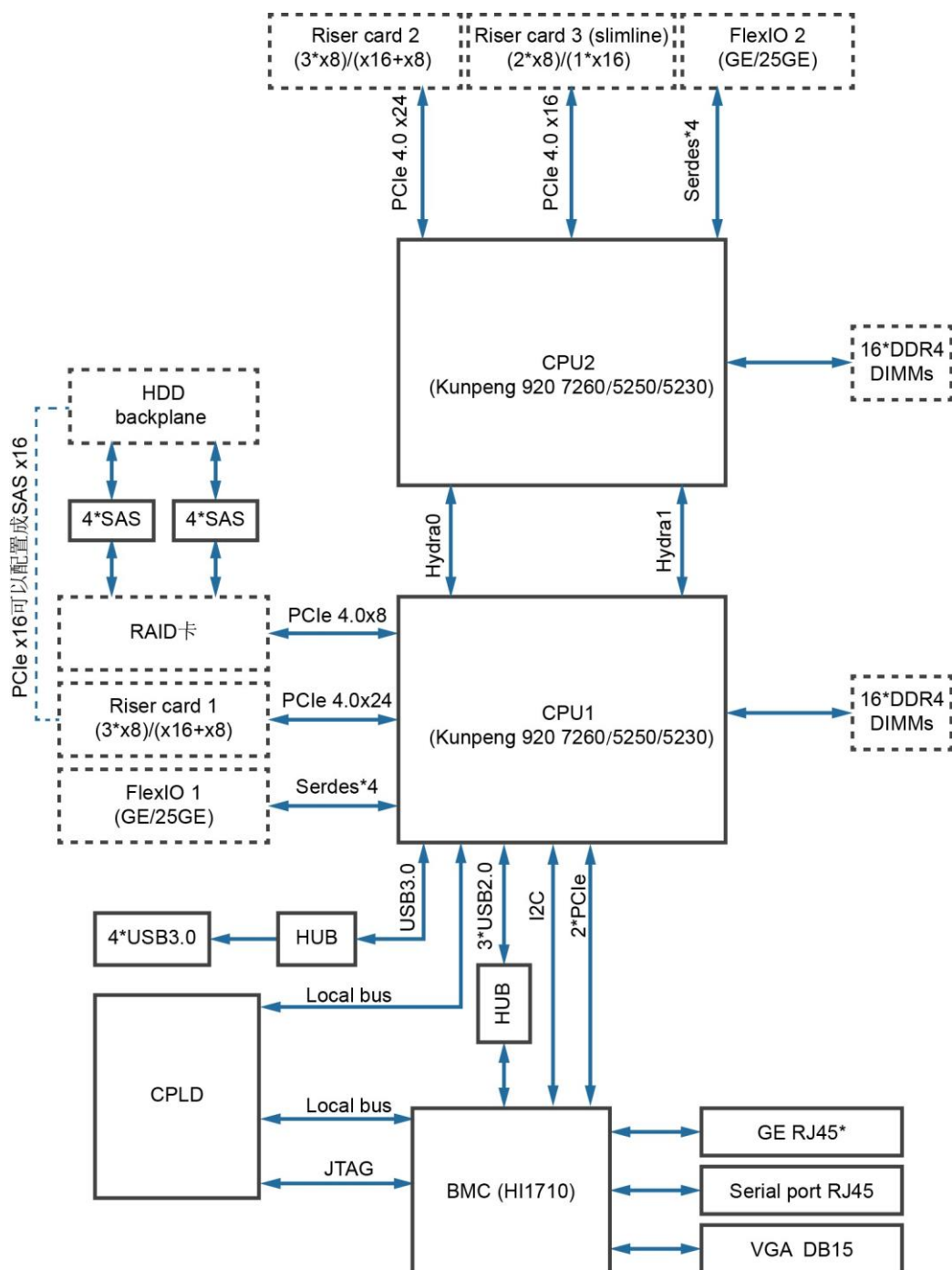
图 1-4 R2232A 逻辑结构（配置鲲鹏 920 7260、5250 或 5230 处理器）
