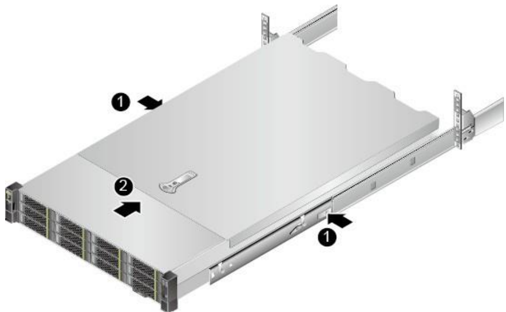
图 5-13 将服务器推入抱轨
